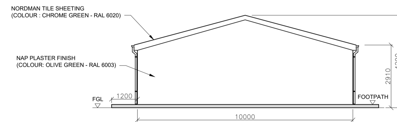
ELEVATION VIEW B SCALE: 1:100
