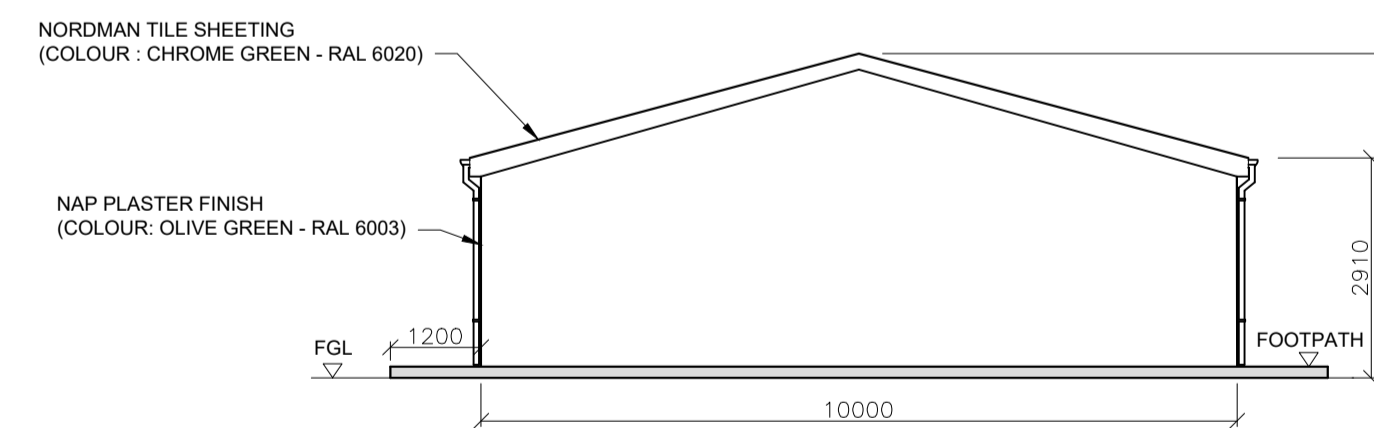
ELEVATION VIEW D SCALE: 1:100
